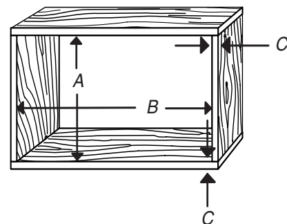
A. 16" (40,6 cm) + 2 x C B. 22 \frac{5}{8} " (57,5 cm) + 2 x C
