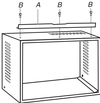
A. Canal superior B. Tornillos Phillips de cabeza de cono achatado #10 - 12 x \frac{3}{8} "
