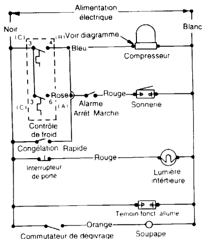
DIAGRAMME DE CABLEAGE
