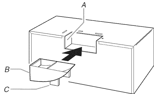
A. Lumbra de escape del horno de microondas B. Lumbra de escape del desviador de aire (extremo abierto) C. Patas del desviador
