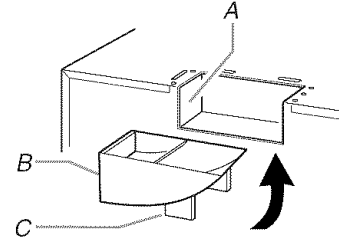
A. Lumbra de escape del horno de microondas B. Lumbra de escape del desviador de aire (extremo abierto) C. Patas del desviador
