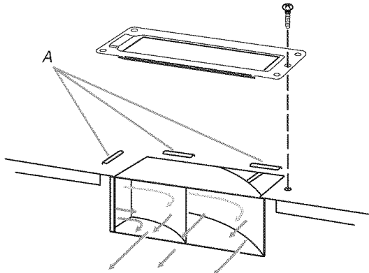
A. Lengüetas de sujeción
