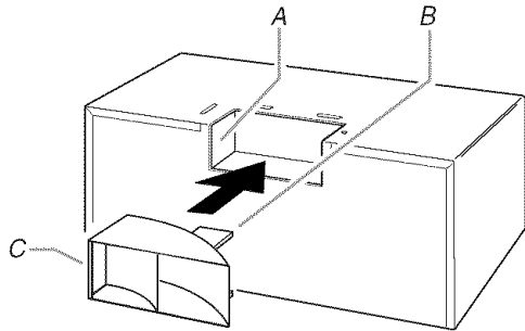
A. Lumbra de escape del horno de microondas B. Patas del desviador C. Lumbra de escape del desviador de aire (extremo abierto)
