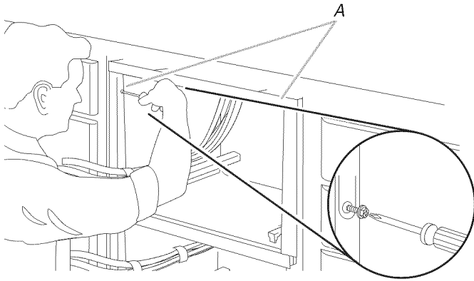
A. Sujete la lavavajillas a los soportes de montaje laterales del armario.
