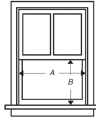
A. 27" mín. (68,6 cm) B. 16 1/4" mín. (41,3 cm)
