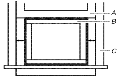
A. Repisa de la ventana B. Gabinete vacío C. Canal de la ventana
