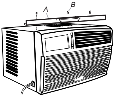
A. Canal superior B. Tornillo de cabeza plana #10 x \frac{3}{8} "
