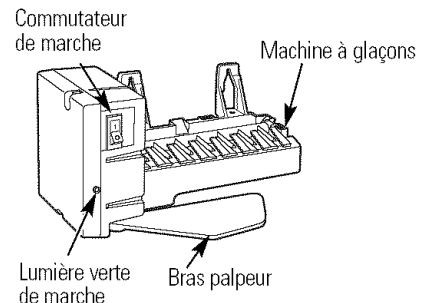
Modèle à commutateur de marche
