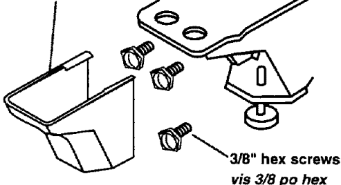
bottom hinge cover couvercle de la charnière inférieure
