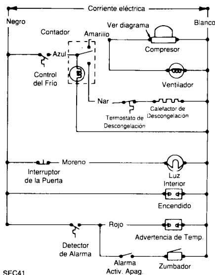
DIAGRAMA DE CABLEADO
