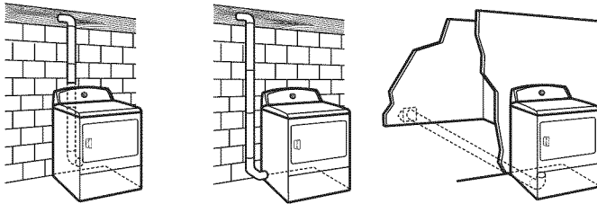
A. Instalación estándar con ventilación en la parte posterior B. Instalación de ventilación lateral a la izquierda o a la derecha C. Instalación con ventilación por la parte inferior
