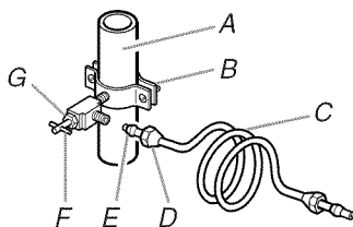
A. Canalisation d'eau froide B. Bride de tuyau C. Tube en cuivre D. Écrou de compression E. Bague de compression F. Robinet d'arrêt G. Vis
