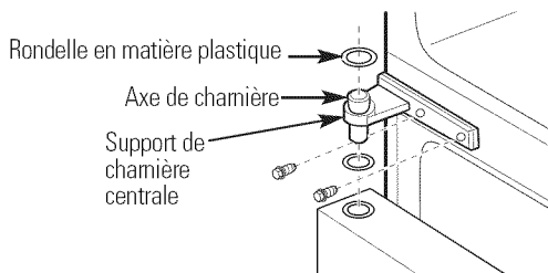
Porte du compartiment réfrigération
